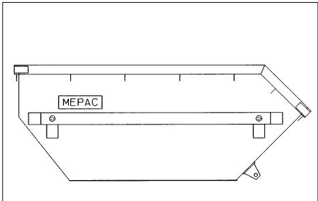
MB 2,5R mit Absetzkippaufnahme
